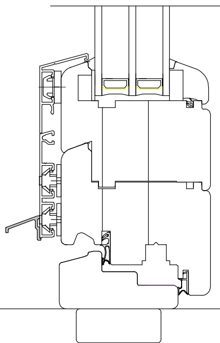
A A-2 Patio Door - Vertical Section
