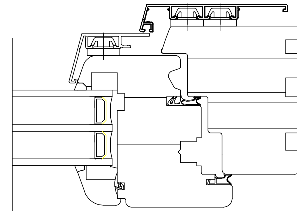
B A-3 Patio Door - Horizontal Section
