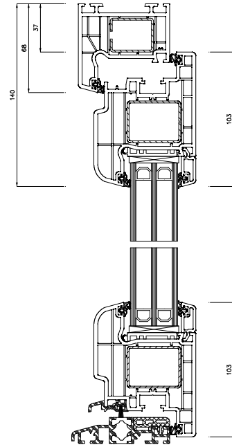
Schnitt S1(5:1)
