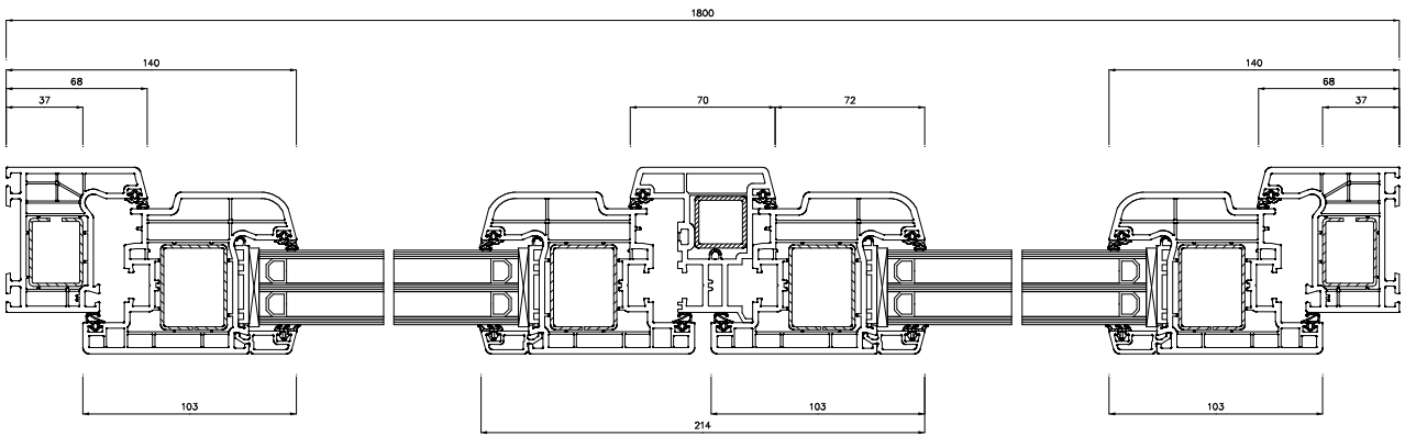
Schnitt S2(5:1)
