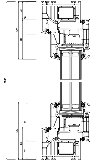
Schnitt S1(5:1)
