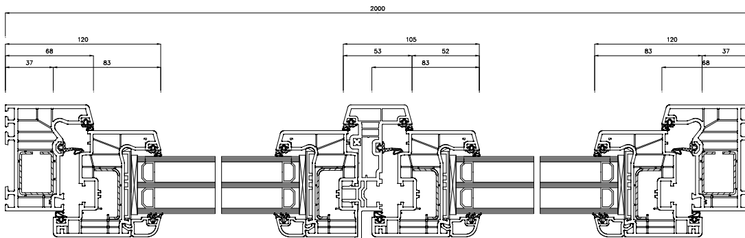
Schnitt S2(5:1)
