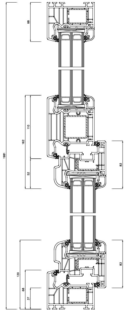
Schnitt S1(5:1)
