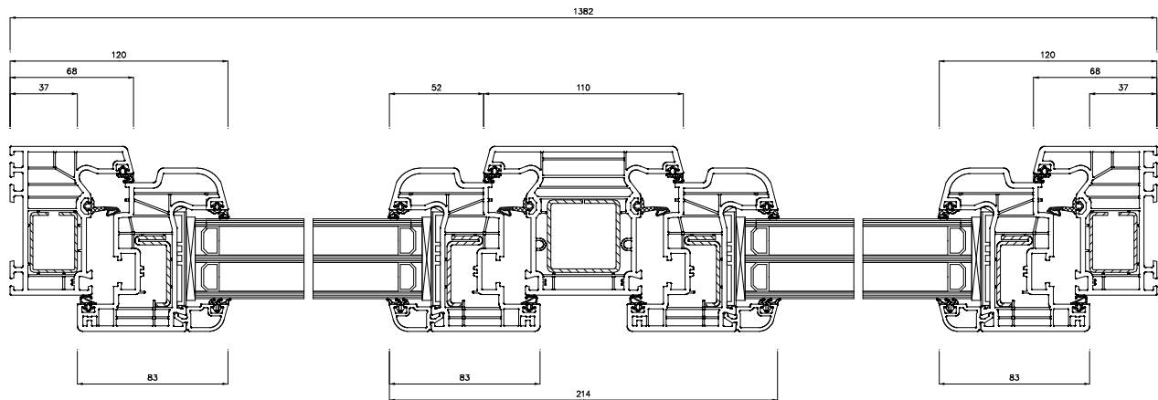
Schnitt S3(5:1)
