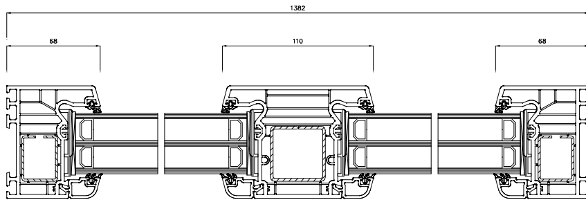
Schnitt S2(5:1)
